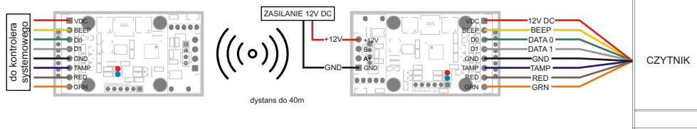
PRZYKŁADOWE PODŁĄCZENIE PRZEDŁUŻACZA Z CZYTNIKIEM I KONTROLEREM SYSTEMOWYM (ZASILANIE Z KONTROLERA SYSTEMOWEGO I ZEWNĘTRZNEGO ZASILACZA)
